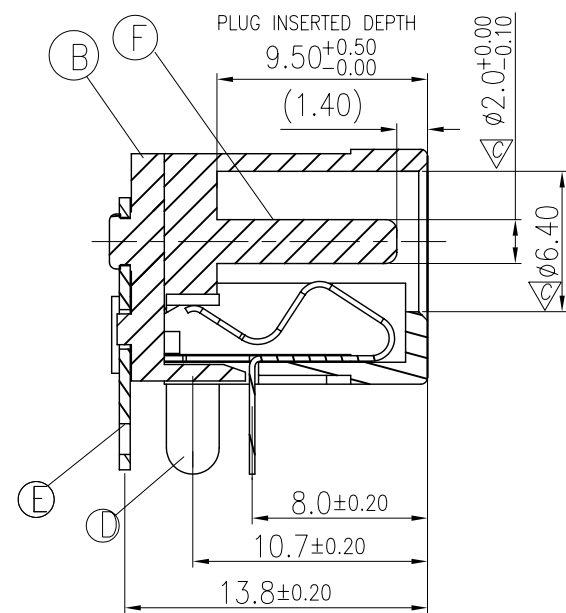
A-A SECTION
