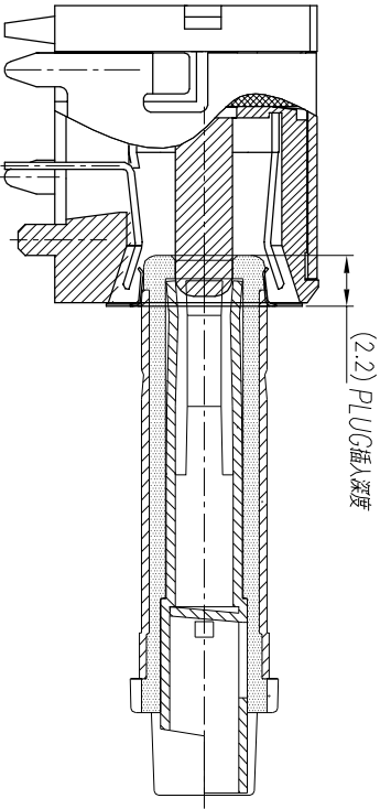
1. GROUND接觸狀態
