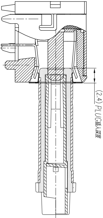
2. 正極 (PIN) 接觸狀態
