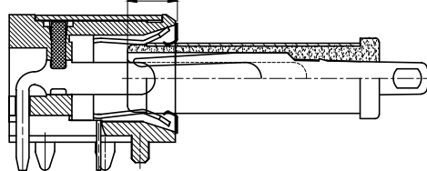
3.SPRING(-)CONTACT
