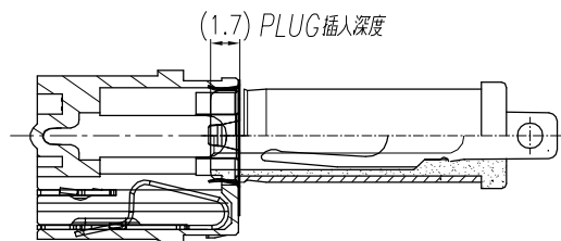
1. 負極端子 (GROUND) 接觸狀態
