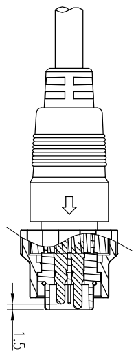
A-A SECTION
