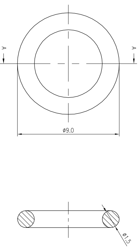
A-A SECTION
