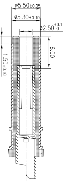
ø5.5 PLUG TYPE(ZDP-G213-B04)
