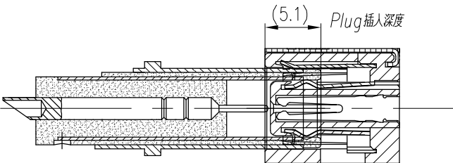
2. 正極接觸狀態
