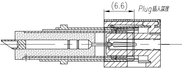
3. SIGNAL 接觸狀態
