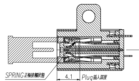
<2.>正極接觸狀態
