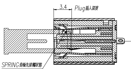
<1.>負極先接觸狀態
