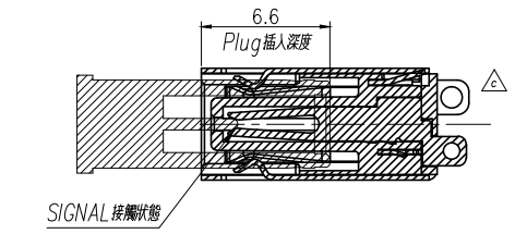
<3.>Signal 接觸狀態
