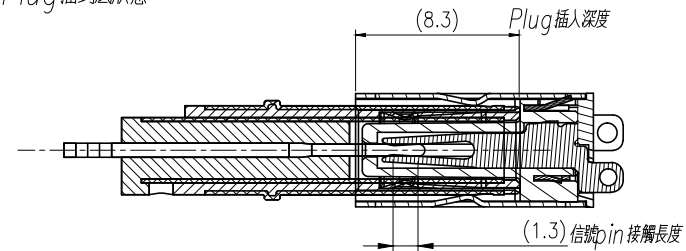
5. Plug 插到底狀態
