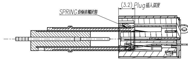
1. SPRING 負極接觸狀態
