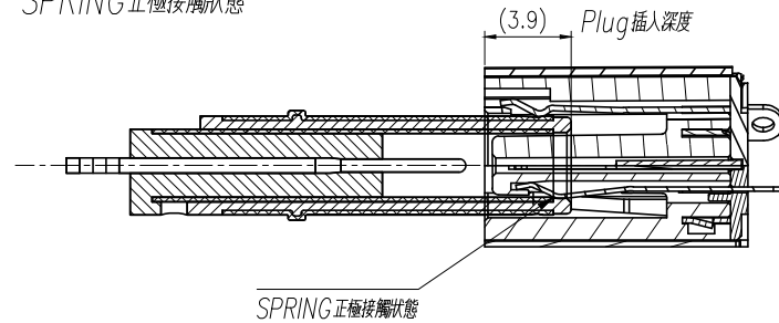
3. SIGNAL PIN 接觸狀態
