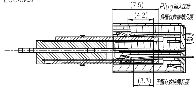
5. Plug 插到底狀態
