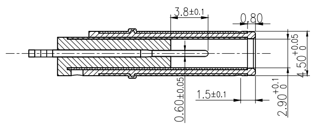
1. SPRING(-) CONTACT
