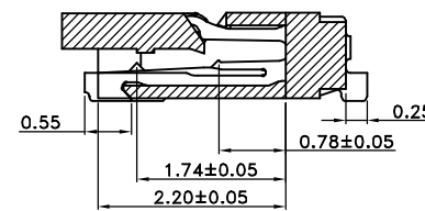
△ Section:A-A Scale 2:1
