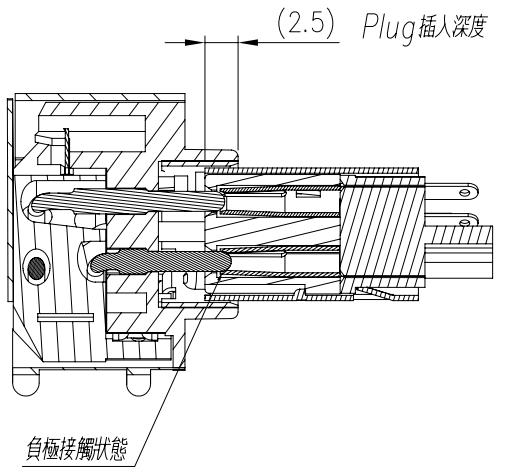
1. 負極接觸狀態
