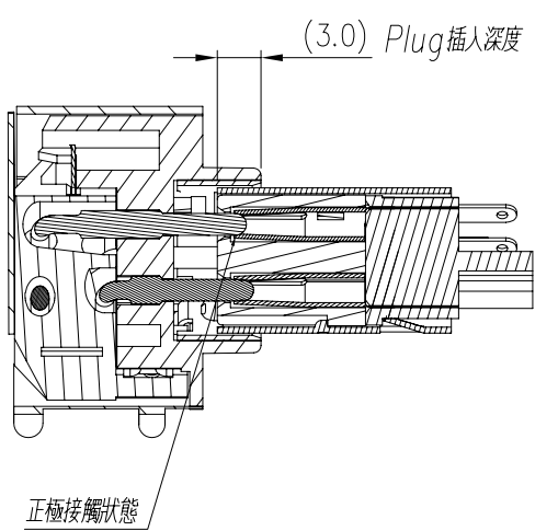
2. 正極接觸狀態
