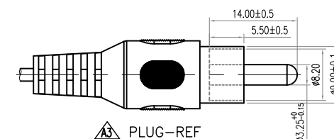
A3 PLUG-REF
