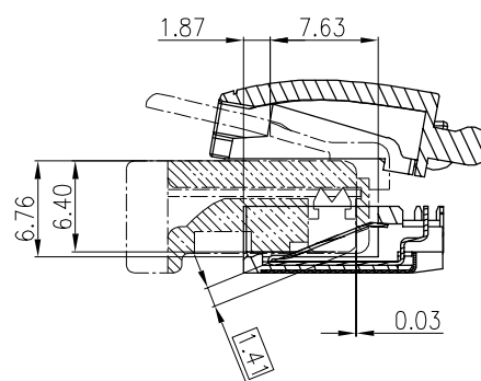
6.40 Plug Worst case 分析
