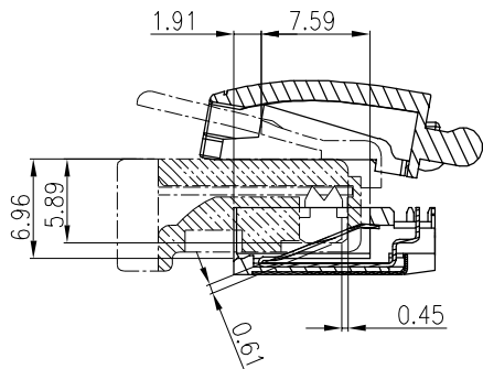
5.89 Plug Worst case 分析
