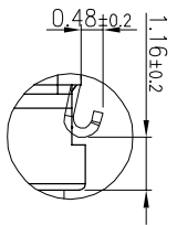
DETAIL:A SCALE:2:1
