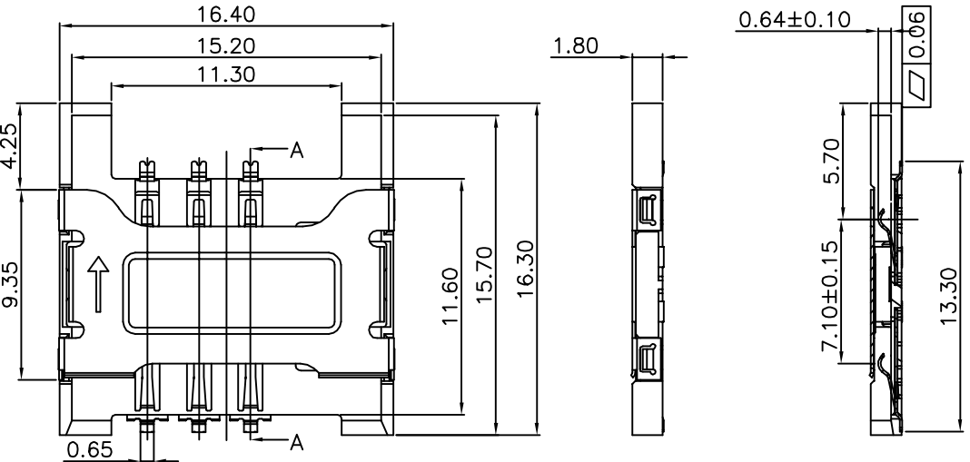
A-A SECTION
