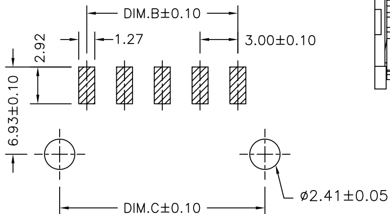
P.C.B. LAYOUT
