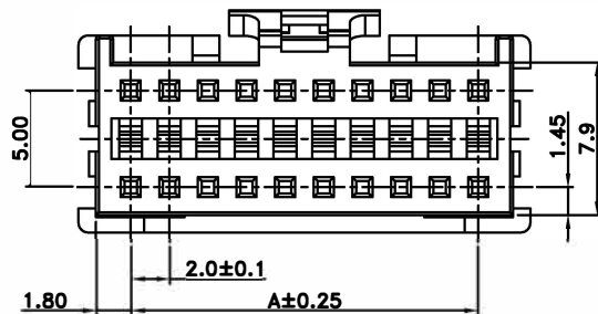
6X2~20X2 PIN
