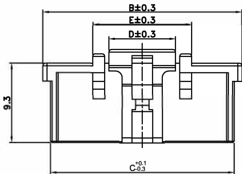
6X2~20X2 PIN
