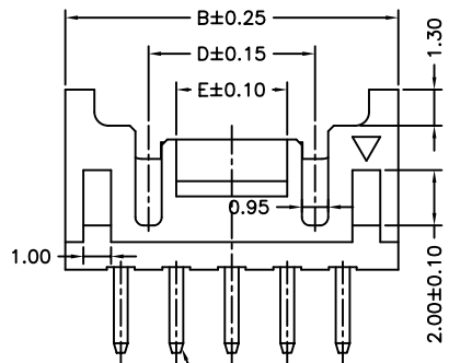
2X05~2X22P
