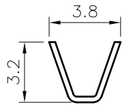
A-A SEC
