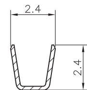
A-A SEC
