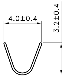
A-A SEC
