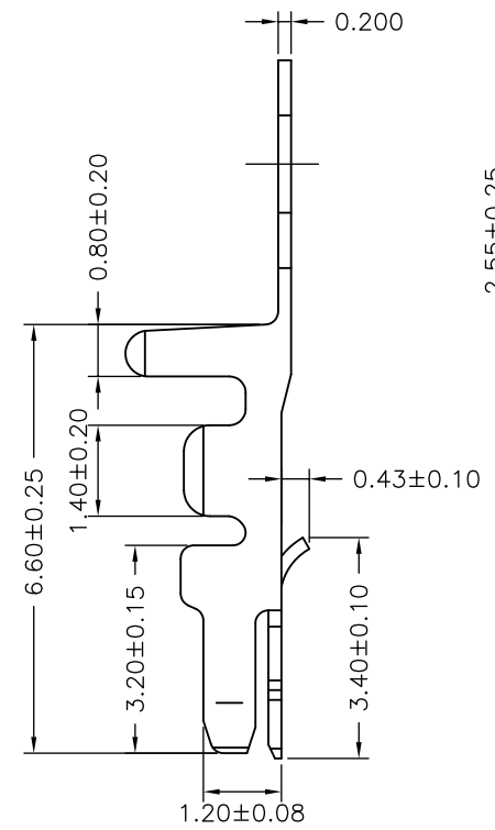
SEC:A-A
