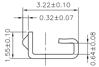
SEC:D-D
