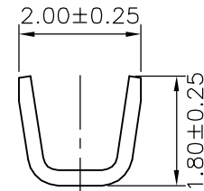
SEC:B-B
